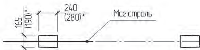
Схема встановлення опори
