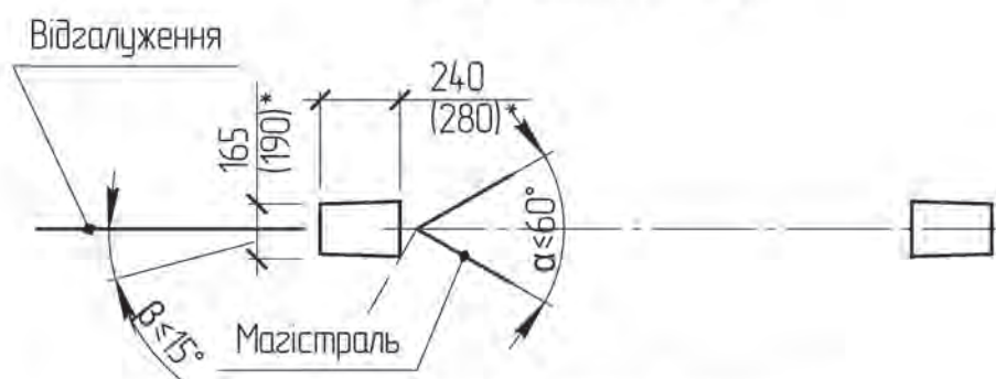
Схема встановлення опори
