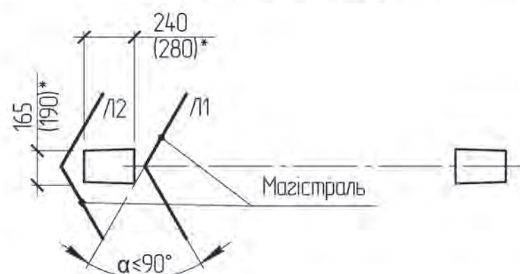
Схема встановлення опори
