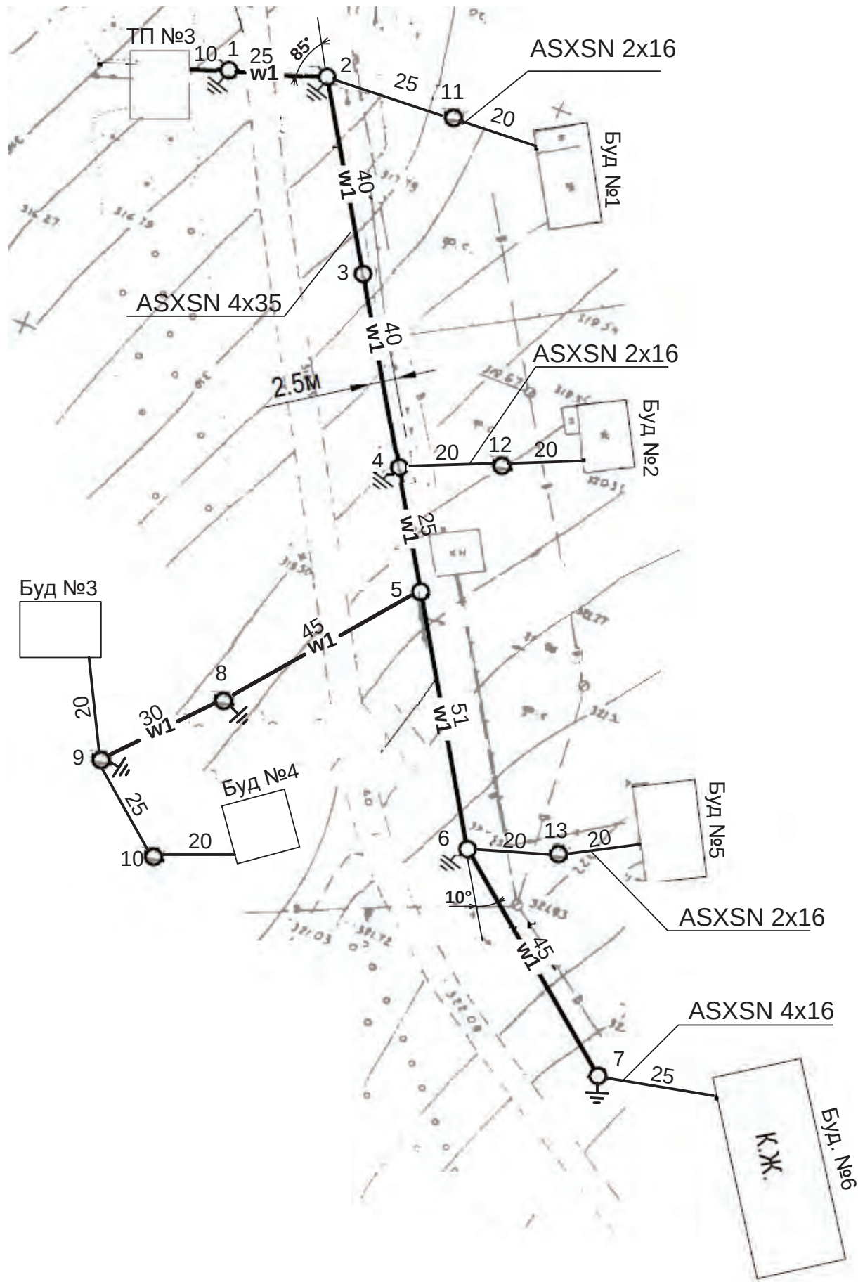
Рисунок 11.1. Приклад розташування опор на трасі ПЛЛ.
