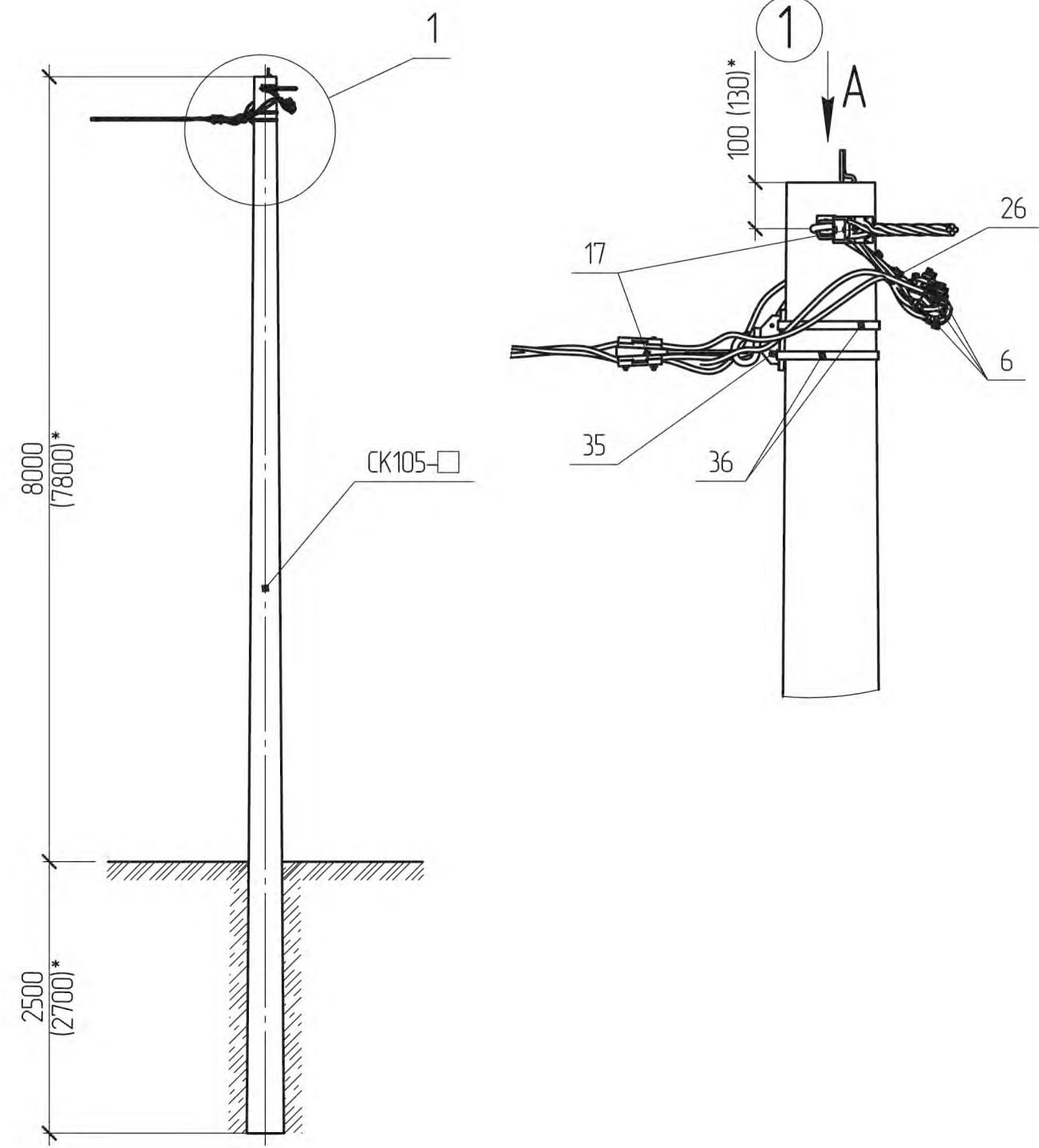
Схема встановлення опори
