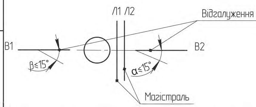
Схема встановлення опори
