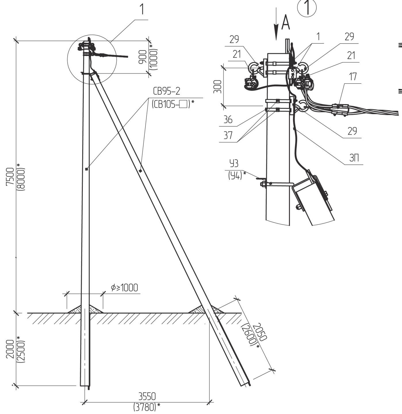
Схема встановлення опори
