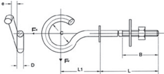
Таблиця 1.12. Вибір гака-долта поз. 31
