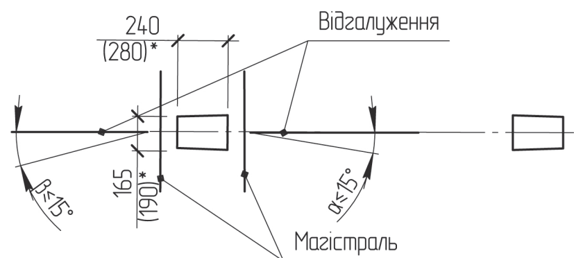
Схема встановлення опори
