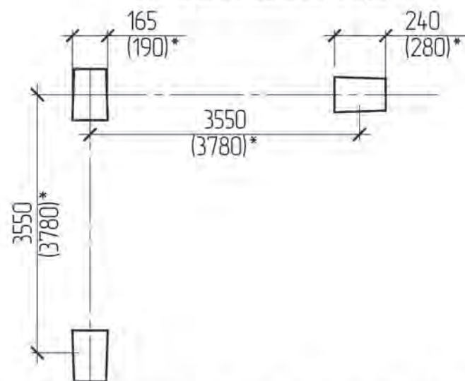
Схема встановлення опори
