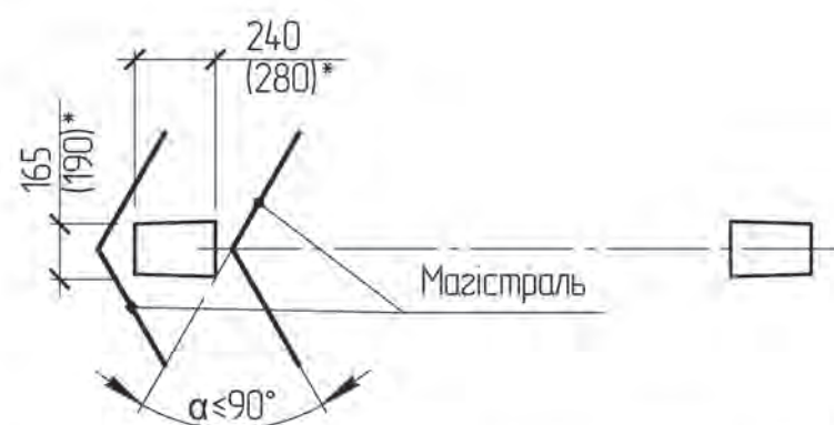
Схема встановлення опори
