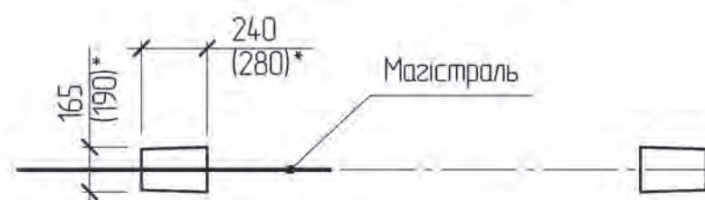
Схема встановлення опори
