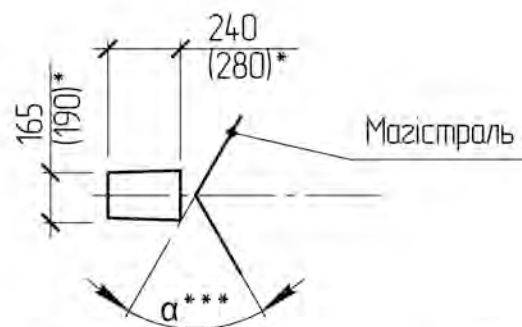
Схема встановлення опори
