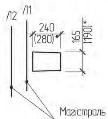
Схема встановлення опори
