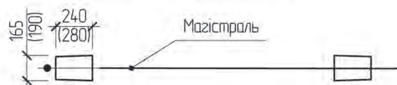
Схема встановлення опори
