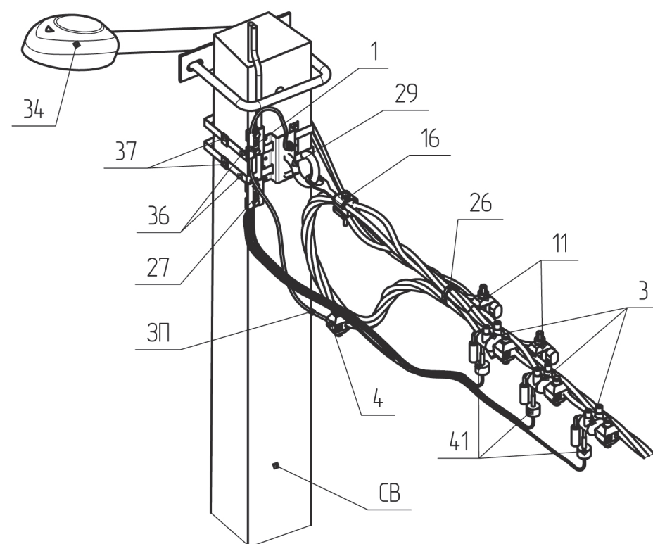
Схема встановлення опори
