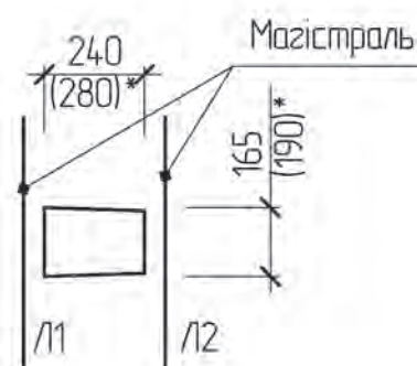
Схема встановлення опори
