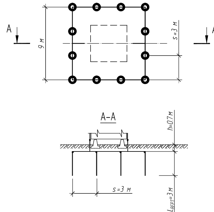
План заземлювального пристрою
