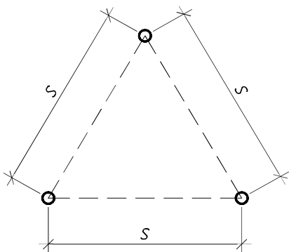
Рис. 3.2 Вертикальні електроди розташовані у формі рівностороннього трикутника
