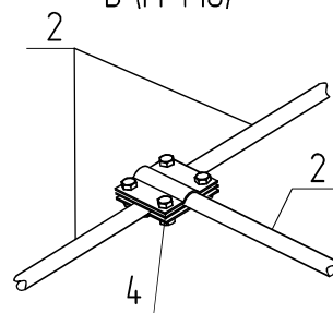
В (М 1:10)
