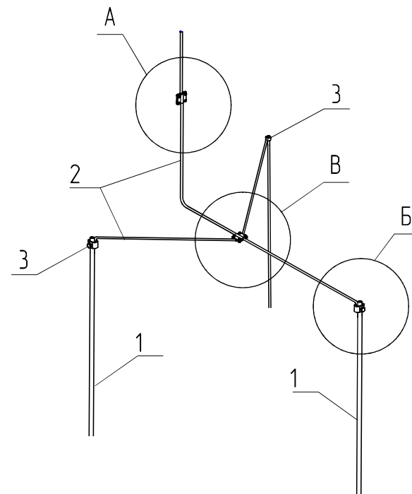
Три вертикальні електроди з'єднані у зірку Загальний вигляд
