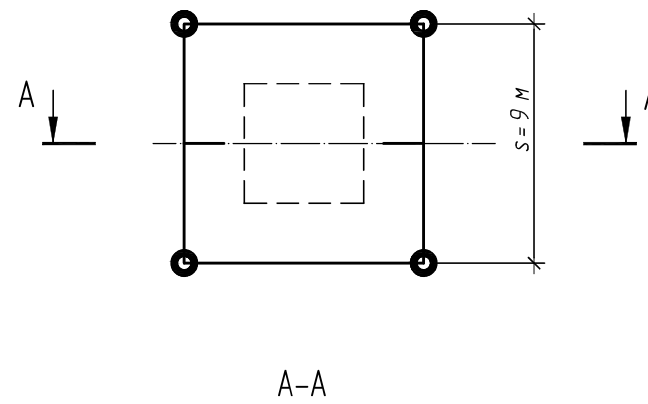
План заземлювального пристрою
