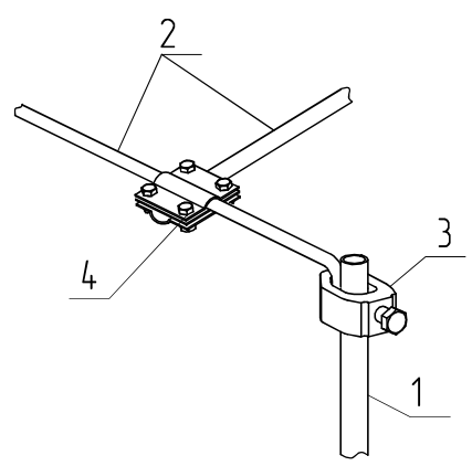
Б (М 1:10)
