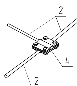
В (М 1:10)
