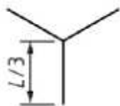
Рис. 3.5 Горизонтальні заземлювачі, з'єднані у зірку під кутом 120
