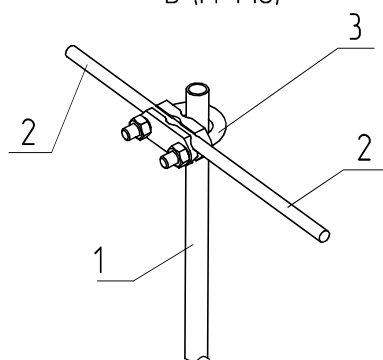
Б (М 1:10)
