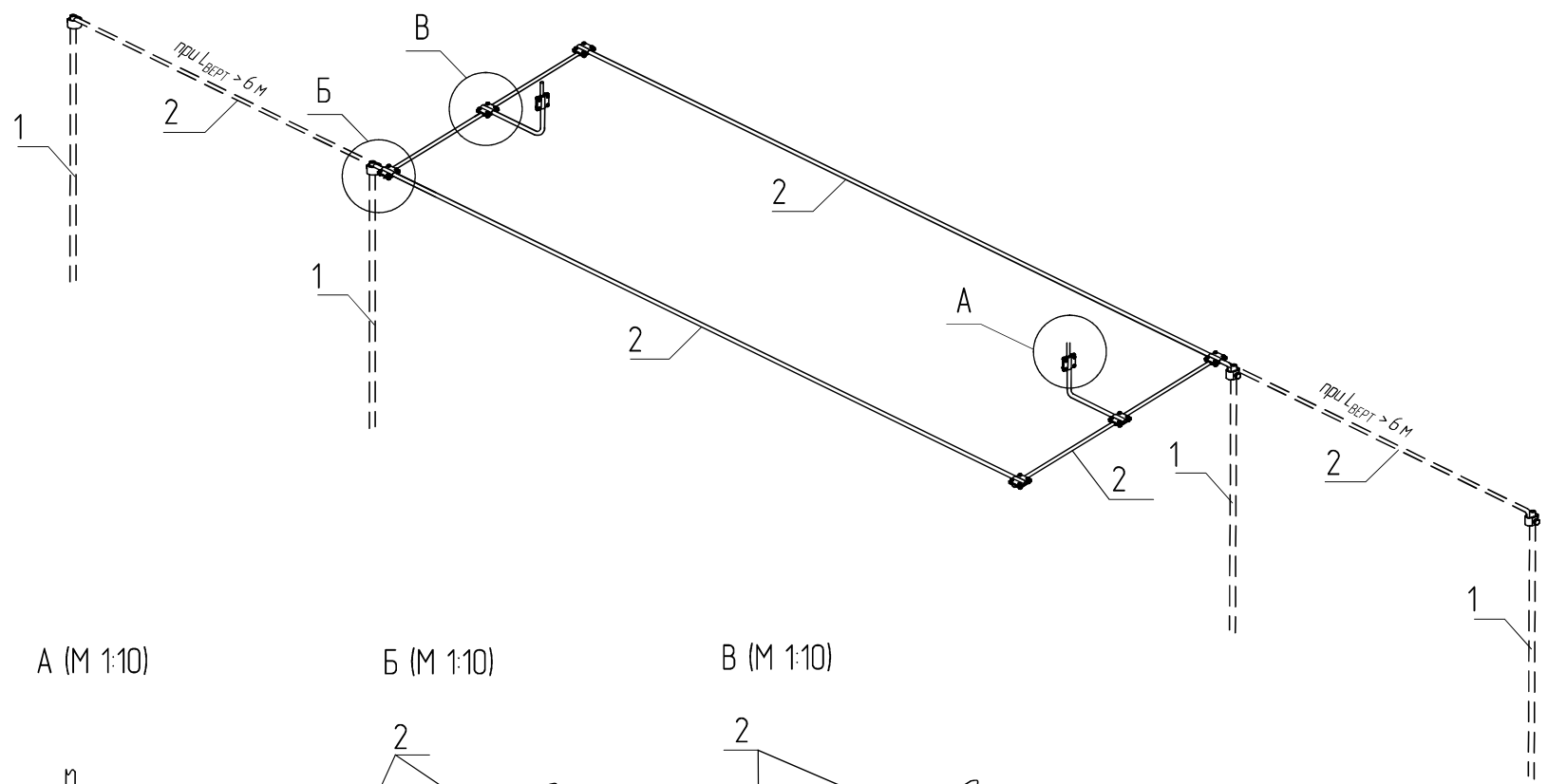
Комбінований заземлювач Загальний вигляд
