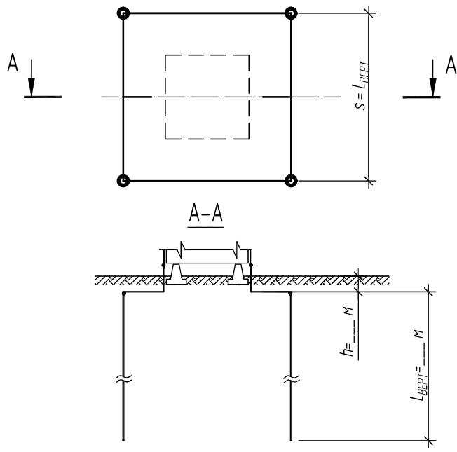
Схема заземлювального пристрою
