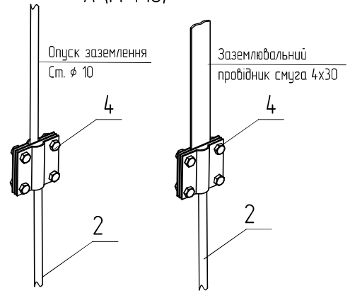
А (М 1:10)
