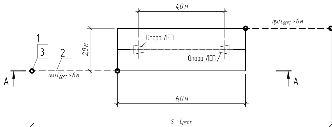
Схема заземлювального пристрою
