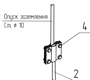
А (М 1:10)
