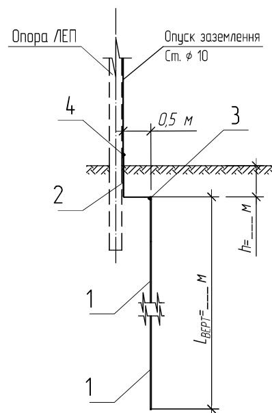
А-А
