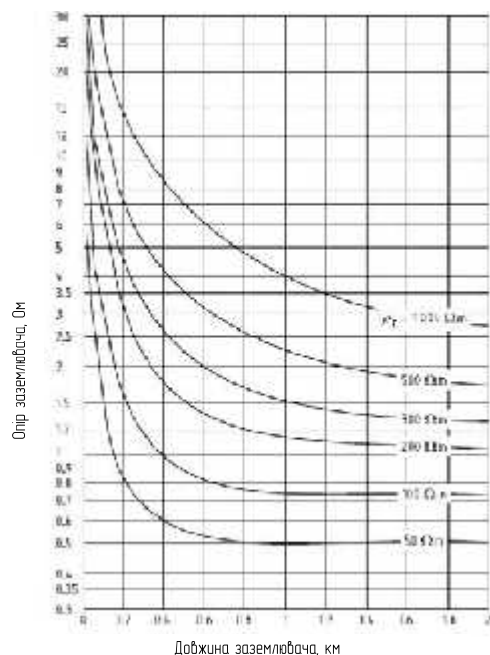
Рис. 3.1 Залежність опору горизонтального заземлювача від його довжини
