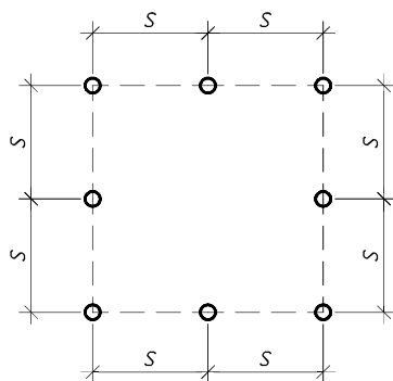
Рис. 3.3 Вертикальні електроди розташовані у формі квадрата
