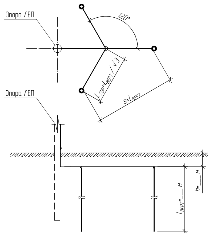
А (М 1:10)
