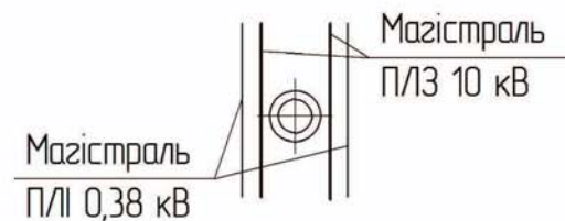
Схема встановлення опори
