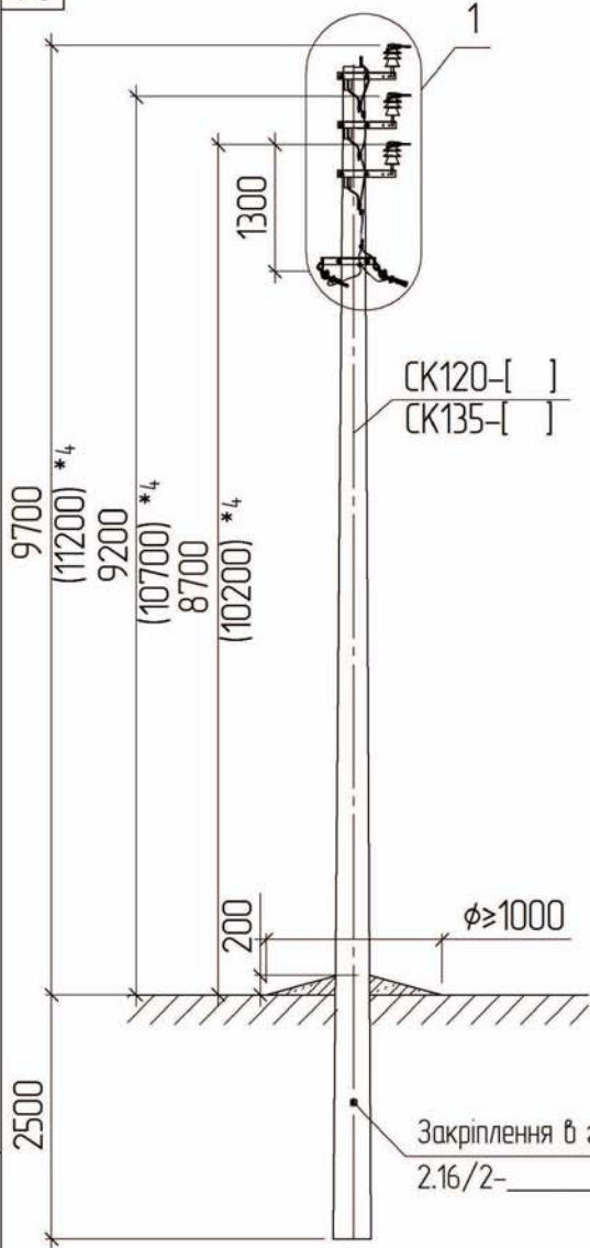
Схема встановлення опори
