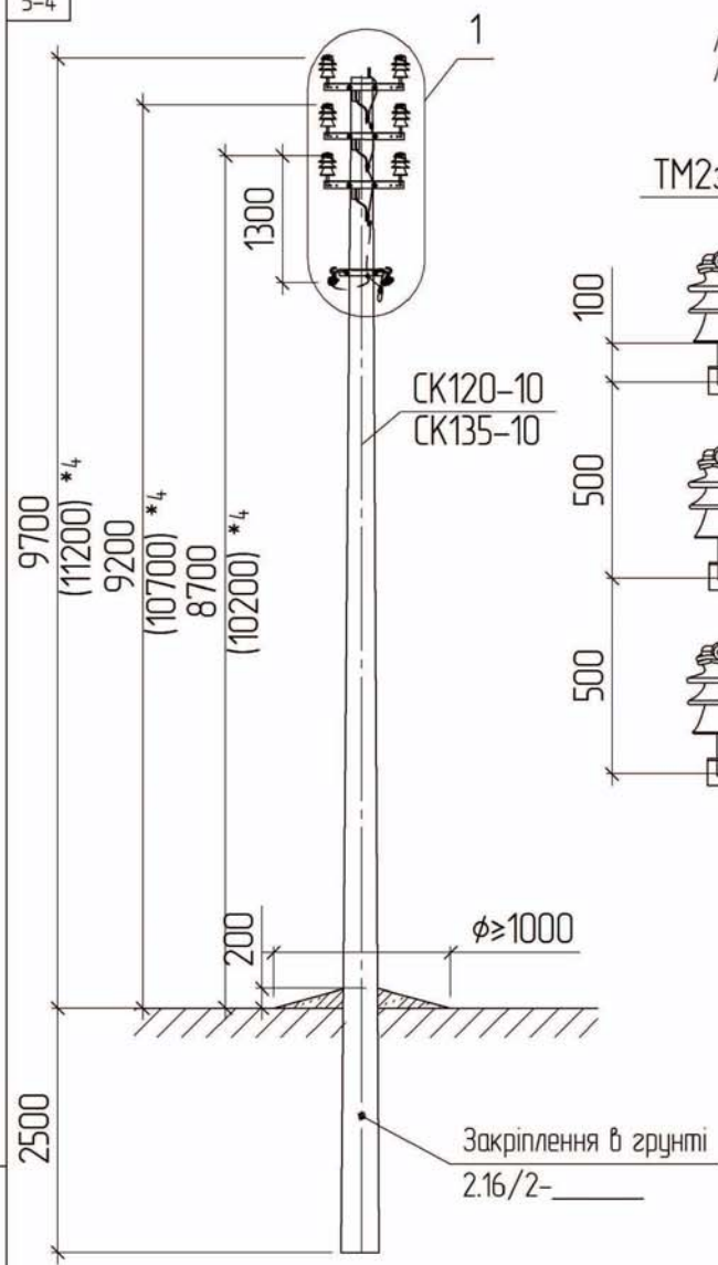
Схема встановлення опори
