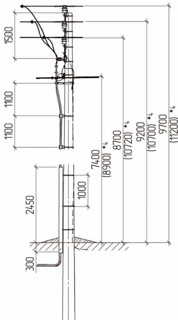
Схема встановлення опори
