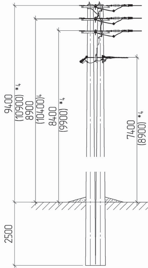
Схема встановлення опори
