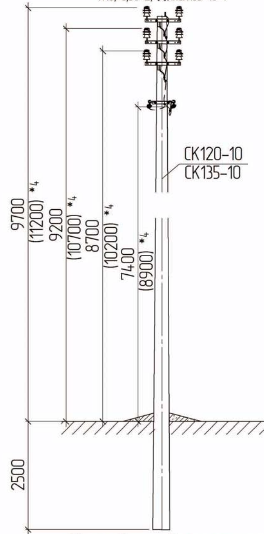
Схема встановлення опори
