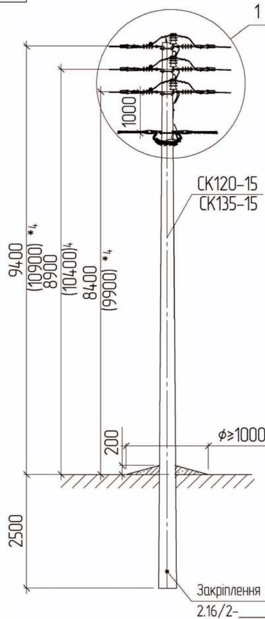
Схема встановлення опори
