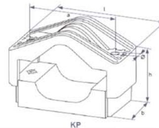
Таблиця 1.21 – Вибір утримувача для 3х одножильних кабелів поз. 24
