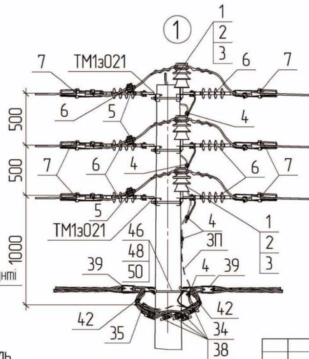
Схема встановлення опори
