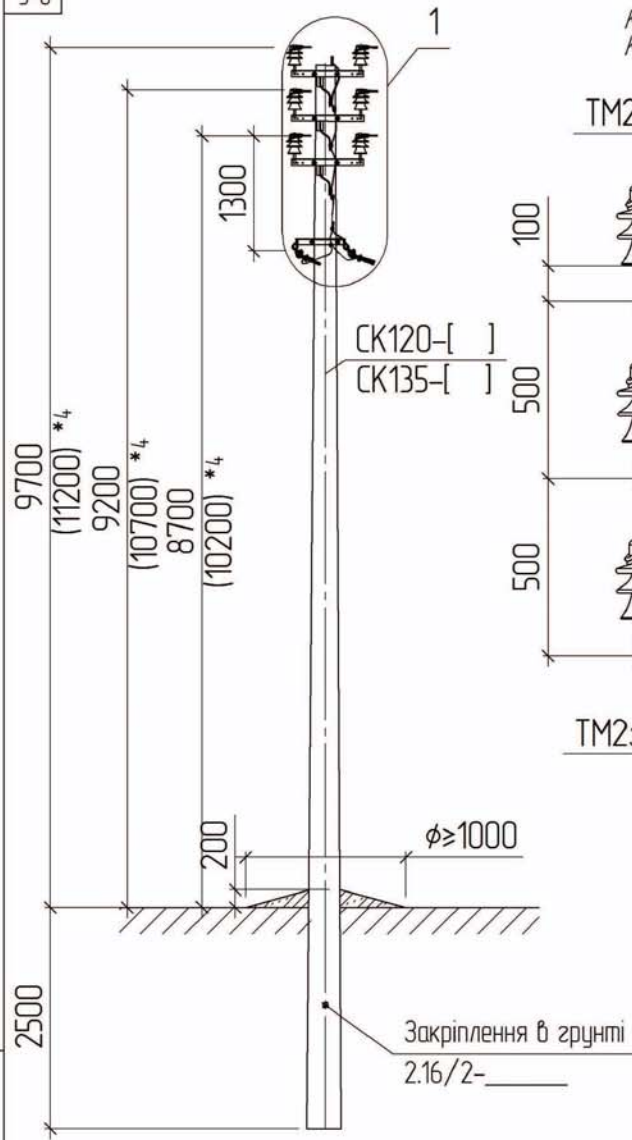
Схема встановлення опори
