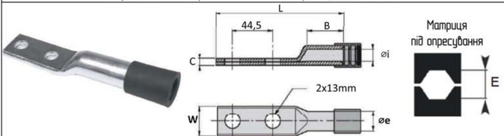
Таблиця 1.20 – Вибір затискача апаратного поз. 23
