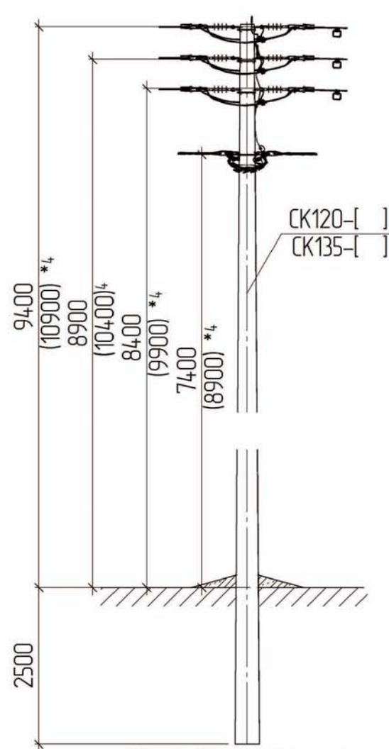
Схема встановлення опори
