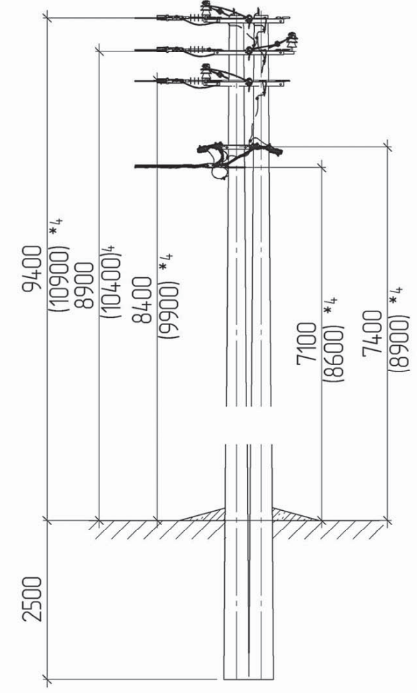
Схема встановлення опори
