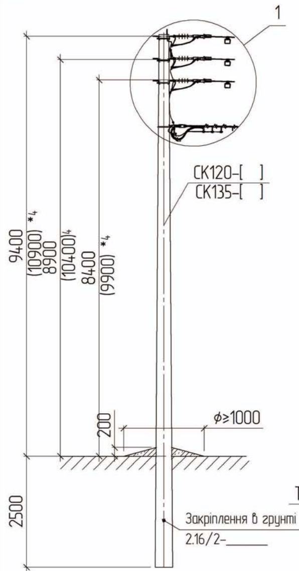
Схема встановлення кінцевої опори
