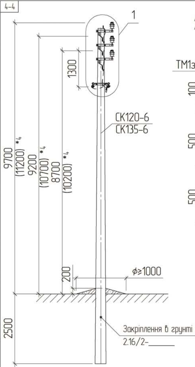
Схема встановлення опори
