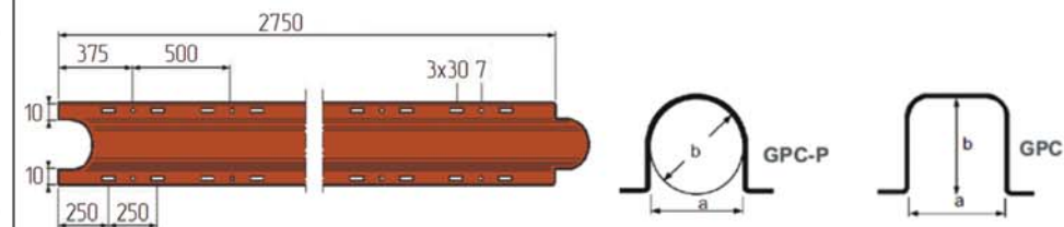
Таблиця 1.10 – Вибір захисної накладки поз. 11 та поз. 45
