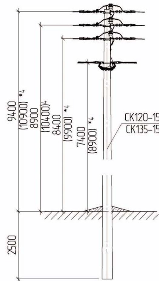
Схема встановлення опори
