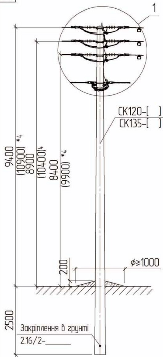
Схема встановлення кінцевої опори
